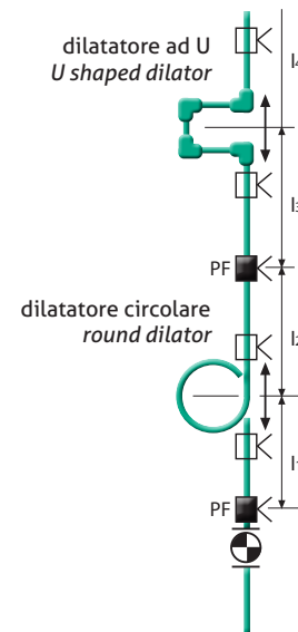
Esempio di compensazione dell'allungamento della tubazione a mezzo di dilatori ad U e circolari.
